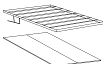
Stelaz z podnośnikami gazowymi oraz dnem, do łóżka 160 x 200 kod: 68 52 23 - 77
