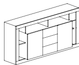
Komoda 2 drzwi, 3 szuflady 172 x 42 x 102 kod: 20 .. 41 - 07
